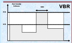
SCR (Sustainable Cell Rate, Sürdürülebilir Hücre İletim Hızı)
